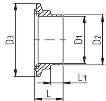
Clamp Nut DIN 11853/3 11866 (B) Nutferrule DIN 11853/3 11866 (B)
