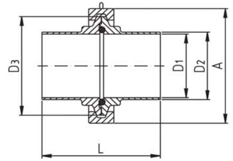
Clamp liner DIN 11864/3 11866 B Bundferrule DIN 11864/3 11866 E
