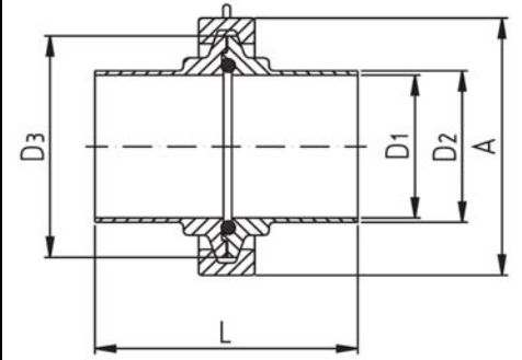
Clamp liner DIN 11864/3 11866 A Bundferrule DIN 11864/3 11866 A
