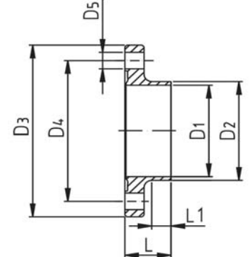
Liner flange DIN 11853/2 ISO 2037 Bundflens DIN 11853/2 ISO 2037
