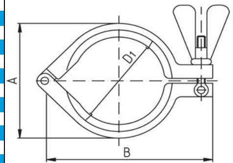
Heavy duty clamp Clampbeugel 2 delig zwaar
