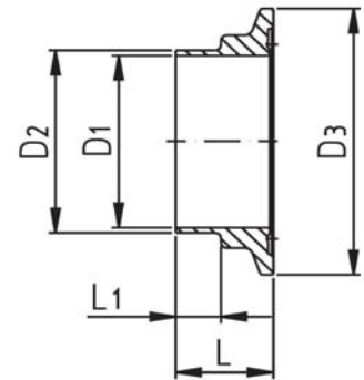
Clamp Nut DIN 11853/3 11850 (2) Nutferrule DIN 11853/3 11850 (2)
