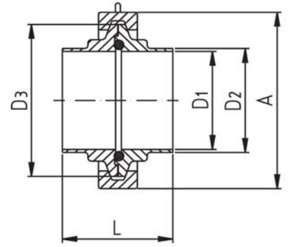
Clamp liner DIN 11853/3 11850 (2) Bundferrule DIN 11853/3 11850 (2)
