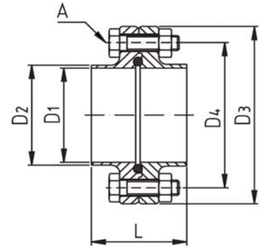
Nut flange DIN 11853/2 ISO 2037 Nutflens DIN 11853/2 ISO 2037
