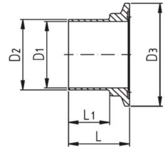
Clamp Nut DIN 11864/3 11866 A Nutferrule DIN 11864/3 11866 A
