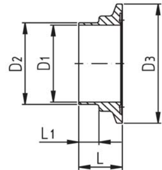
Clamp liner DIN 11853/3 11866 (B) Bundferrule DIN 11853/3 11866 (B)
