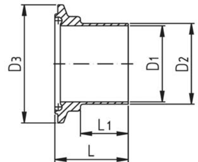
Clamp Nut DIN 11864/3 11866 E Nutferrule DIN 11864/3 11866 B
