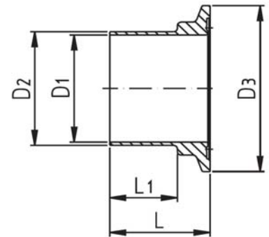
Clamp Nut DIN 11864/3 11866 E Nutferrule DIN 11864/3 11866 B
